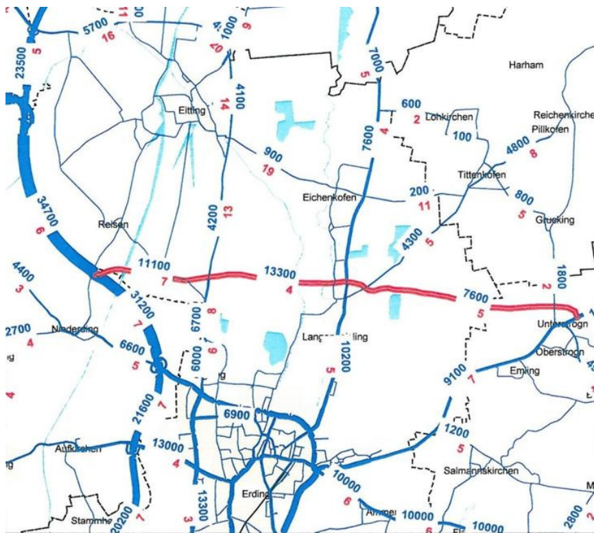
Abbildung 2: Verkehrsbelastungen (Kfz/24h) Prognose 2025 Wahltrasse Süd 2 mit Schwerverkehrsanteilen in Prozent (rot)
