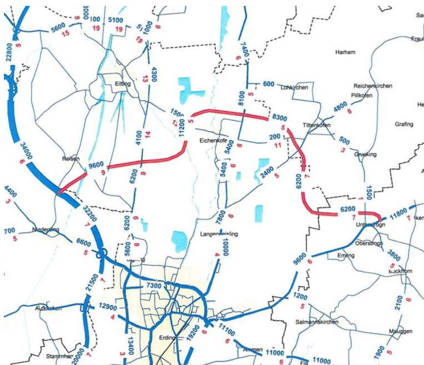
Abbildung 3: Verkehrsbelastungen (Kfz/24h) Prognose 2025 Wahltrasse Mitte 3 mit Schwerverkehrsanteilen in Prozent (rot)
